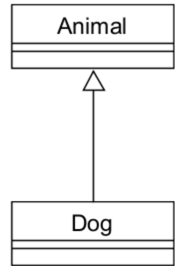
继承关系
