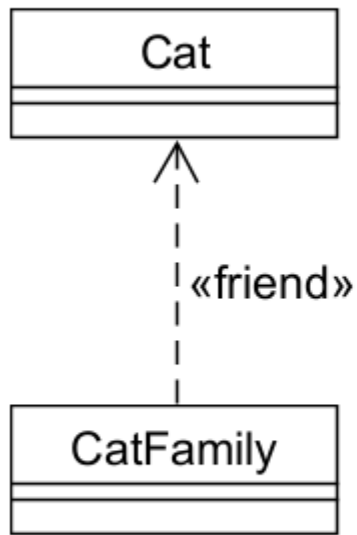
友元关系
